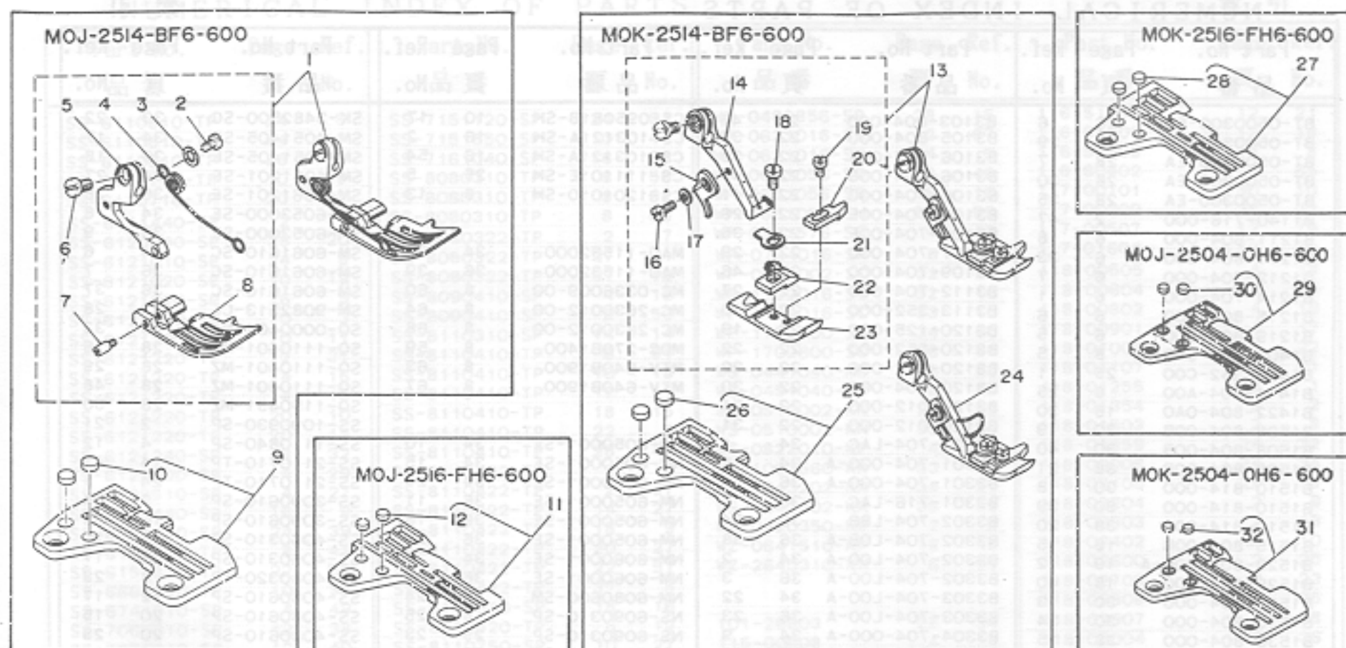
MOJ-2514-BF6-600
